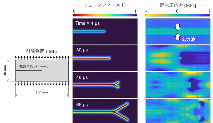
高速進展モードIき裂の分岐挙動の数値シミュレーション
