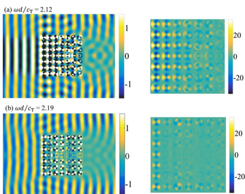
フォノンニック結晶平板における曲げ波の遮断（多数の散乱体の共振を利用）
