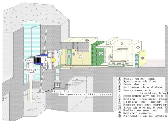
原子炉を利用した照射システム(KUR 重水設備)
