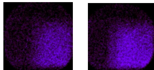
減速材表面の冷中性子分布。左がポリエチレン前置減速材のない場合、右がある場合。前置減速材がある方が冷中性子強度が強い。
