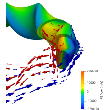
図2：電磁流体平衡における Pfirsch-Schlüter 流
