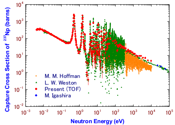
反応断面積の測定例。マイナーアクチニド核種といわれる Np-237 について、その中性子捕獲断面積の新しい測定結果を示している(Present(TOF))。
