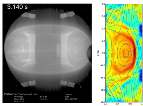
図3：可視光トモグラフィーによる電磁流体平衡の推定
