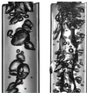
気液二相流
